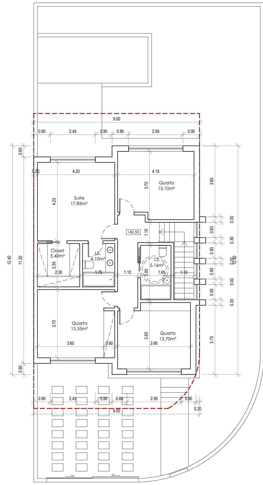
Piso 1
